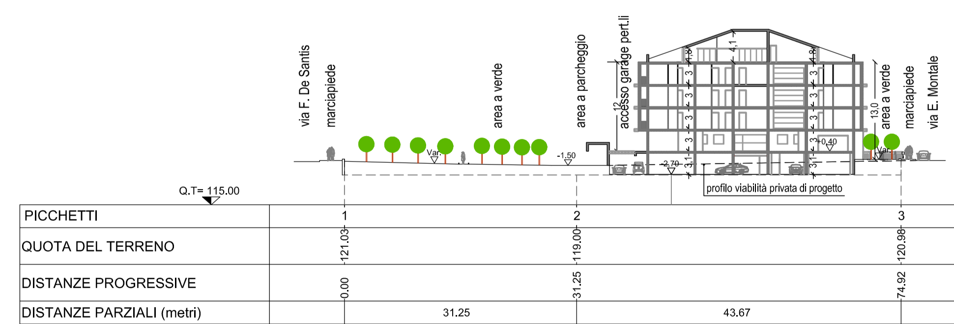
PROFILO 2-2
